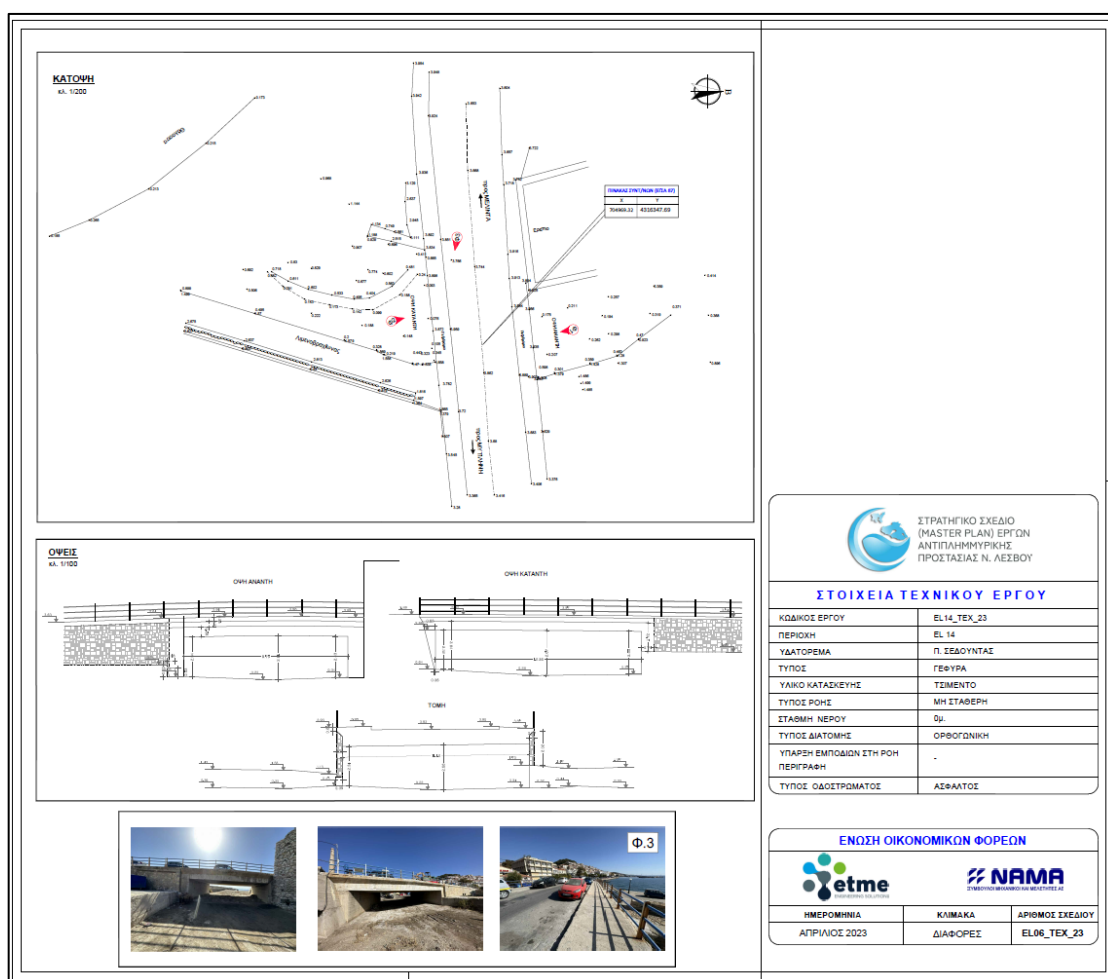
Σχήμα 5. Ενδεικτικό Σχέδιο Αποτύπωσης τεχνικού EL14_TEX_23
