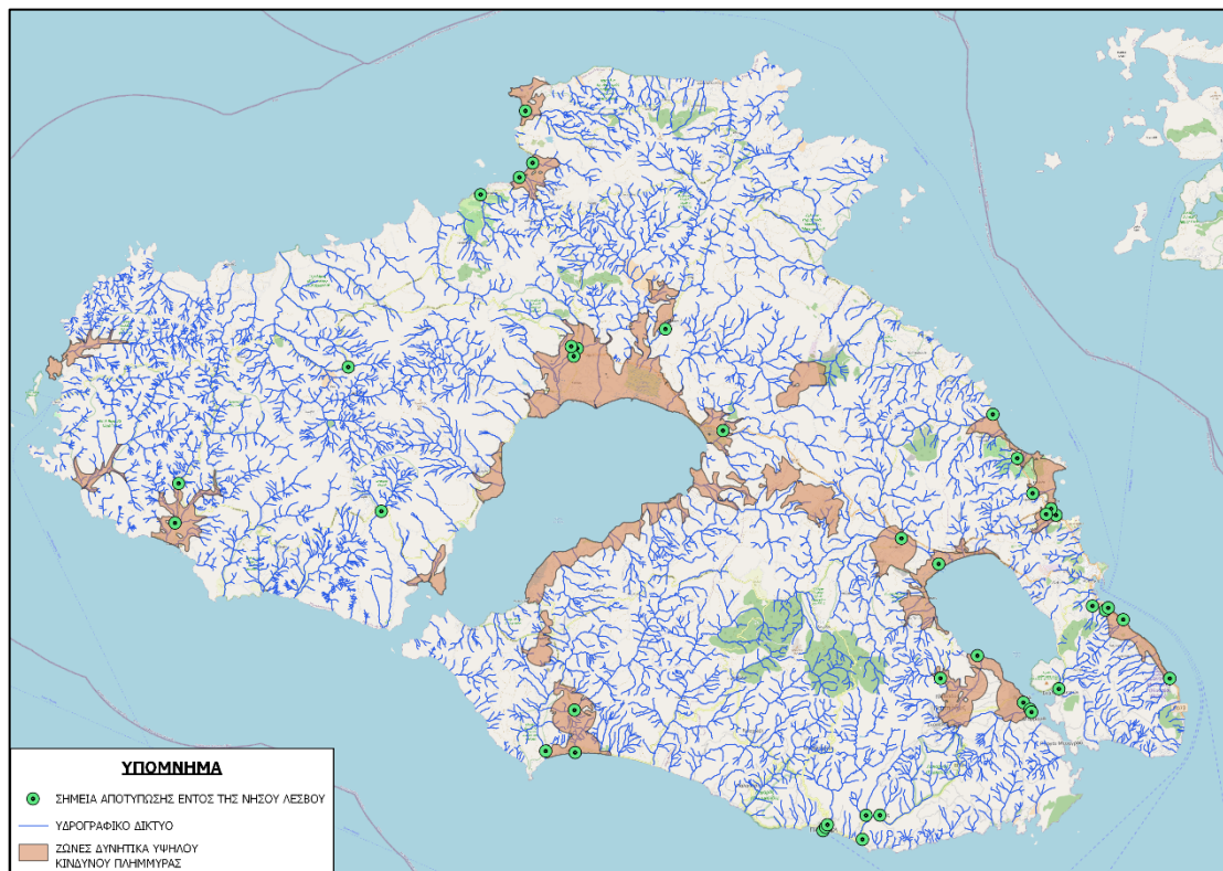
Σχήμα 3. Τεχνικά τα οποία αποτυπώθηκαν εντός της νήσου Λέσβου
