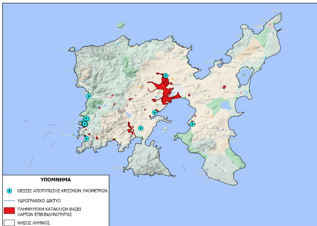
Σχήμα 8. Θέσεις αποτύπωσης κρίσιμων υψομέτρων Νήσου Λήμνου
